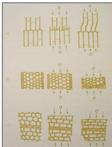
Figura 2 – Mecanismos de deformação da madeira em compressão: (a) axial, (b) radial e (c) tangencial (Rosa, 2003, p. 446).
